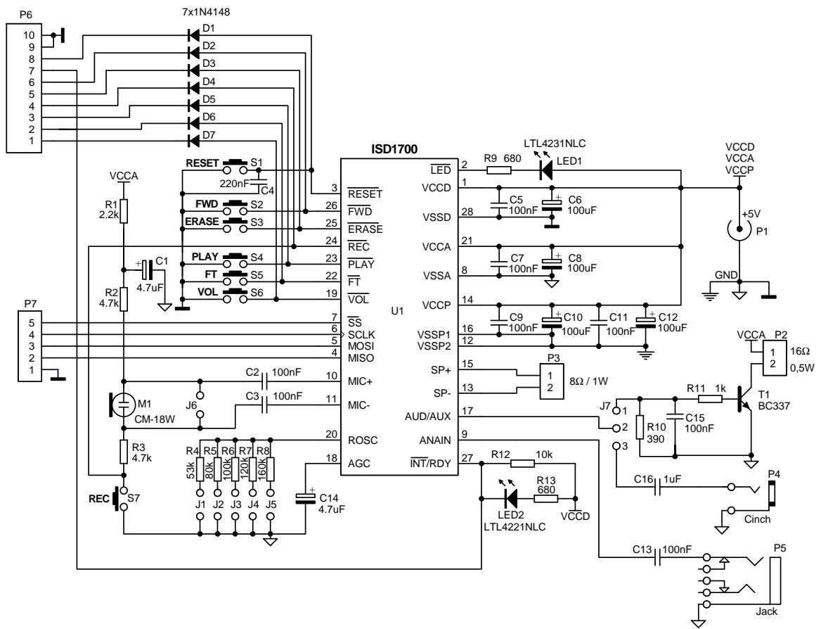
Rys.1. Schemat ideowy modułu MART1700.
