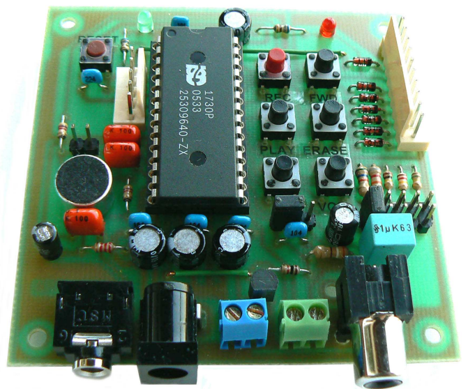
Rys.2. Rozmieszczenie elementów na płycie drukowanej MART1700 (skala 1,2 : 1).
