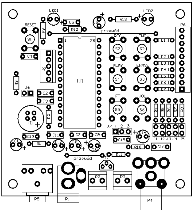
Rys.2. Rozmieszczenie elementów na płycie drukowanej MART1700 (skala 1,2 : 1).
